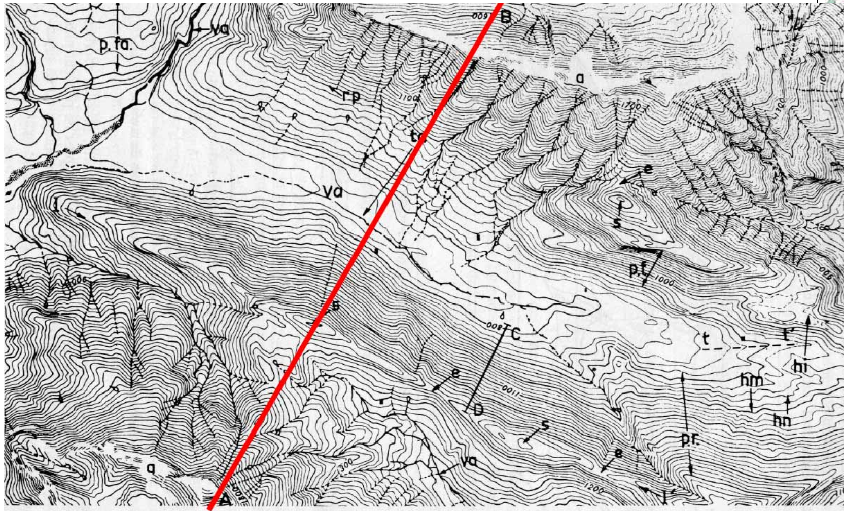
FIG. 8. — Extrait de la feuille d'Albertville (XXXIV-32) 1/50 000 édition orohydrographique.
